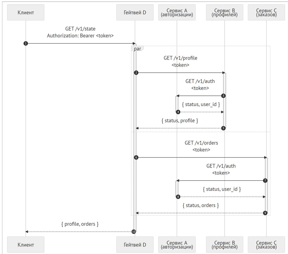
Исходная схема организации микросервисов
