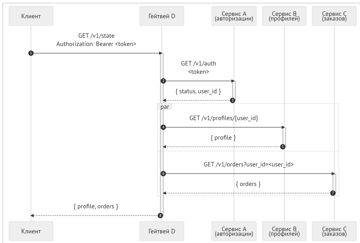
Шаг 1. Явные идентификаторы пользователей
