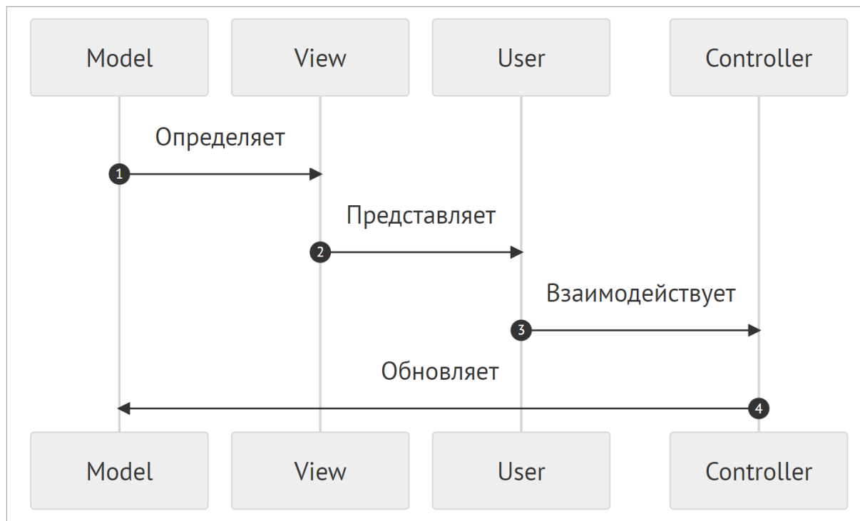
Схема взаимодействия компонентов в MVC
