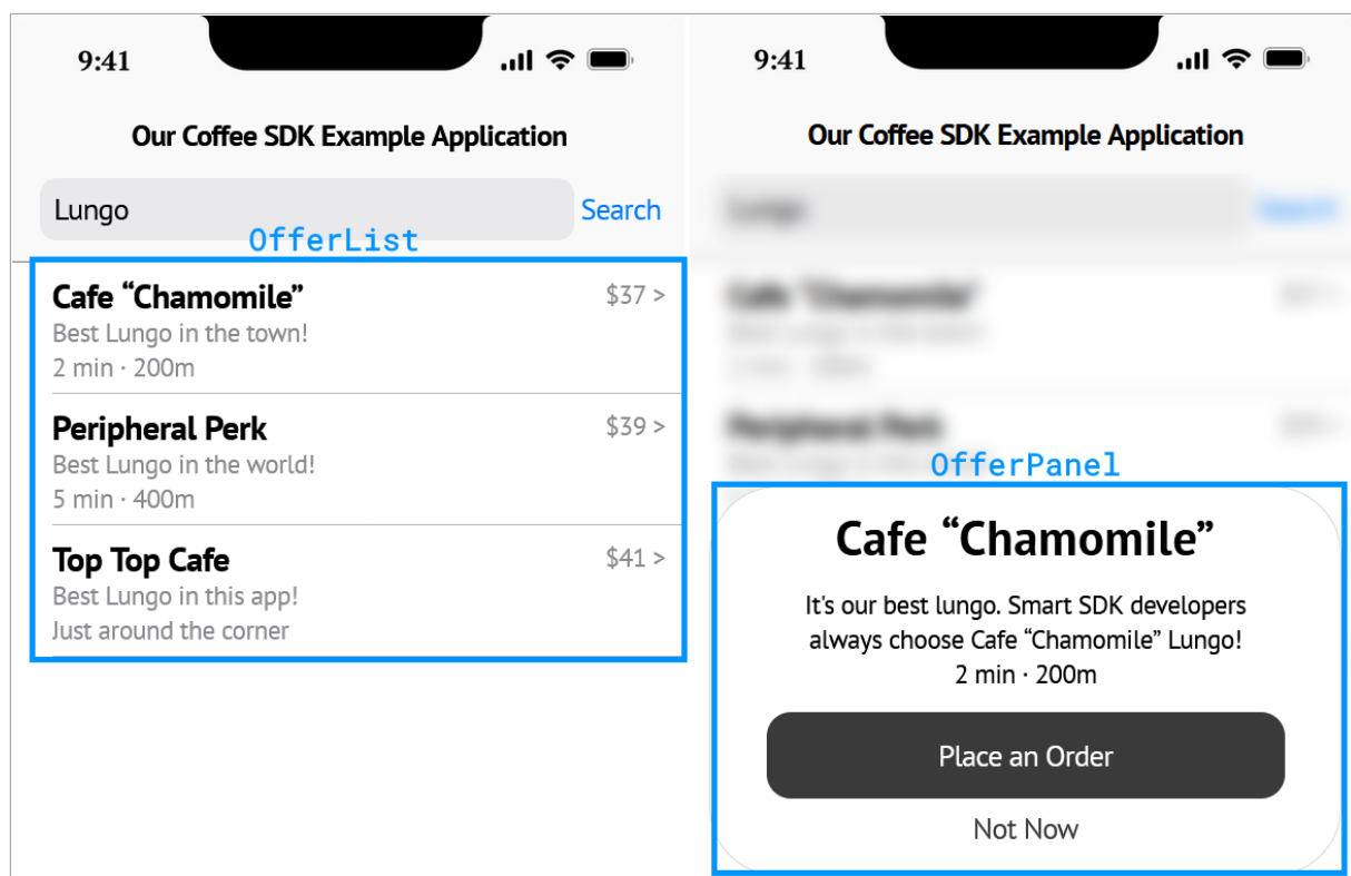
`SearchBox` и его суб-компоненты
