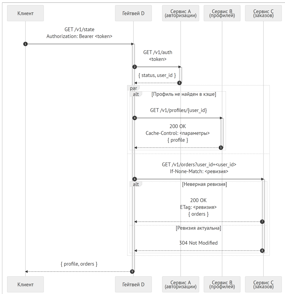
Шаг 2. Добавление серверного кэширования
