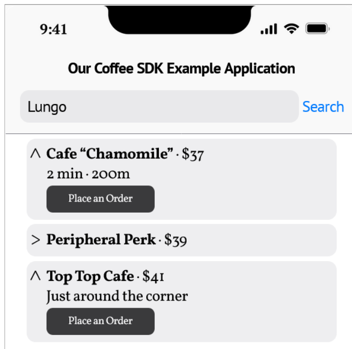
Список результатов поиска, в котором некоторые предложения развёрнуты
